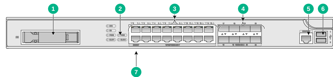
图A-5 设备前视图
