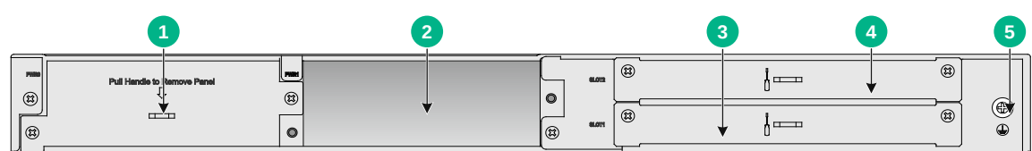
图A-8 设备后视图
