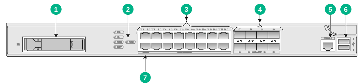
图A-3 设备前视图
