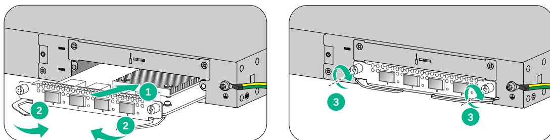
图2-13 安装接口模块
