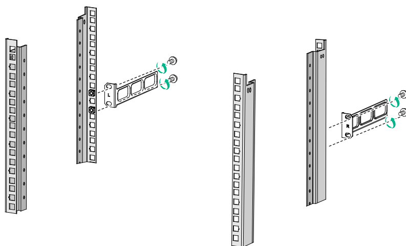
图2-5 安装后挂耳（后挂耳反装）
