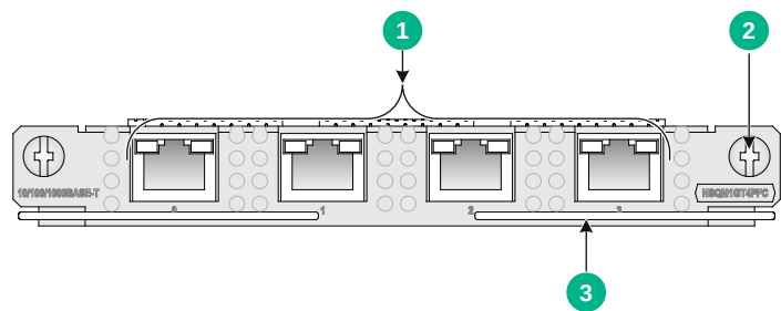
图A-9 NSQM1GT4PFC 接口模块正视图
