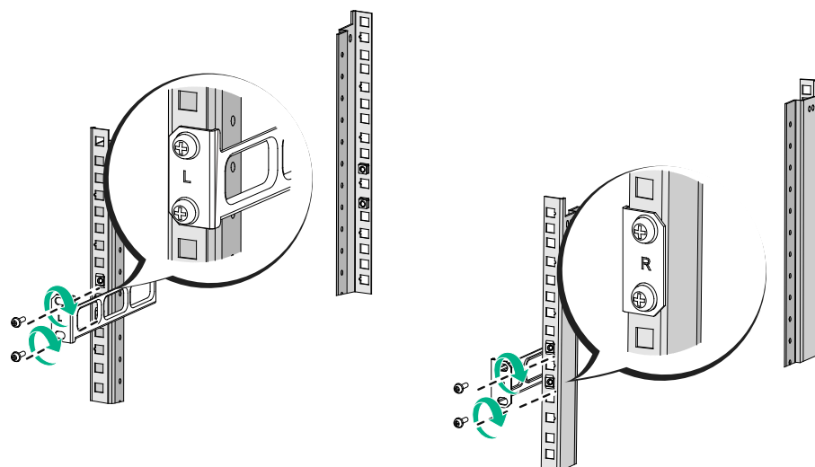
图2-4 安装后挂耳（后挂耳正装）
