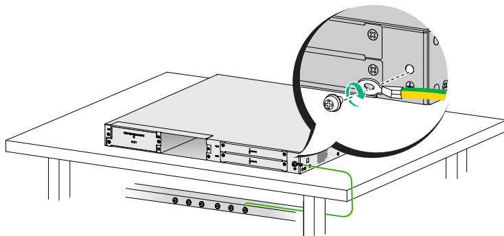
图2-8 通过接地排接地.
