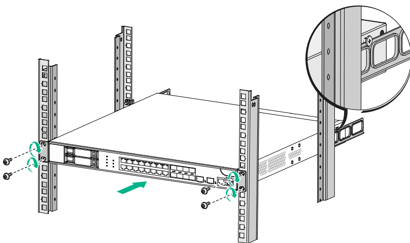
图2-7 安装设备到机柜（后挂耳反装）
