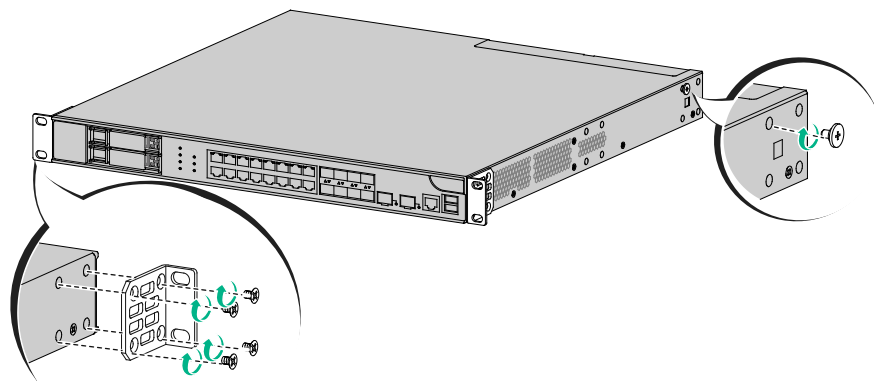
图2-3 安装前挂耳和承重螺钉
