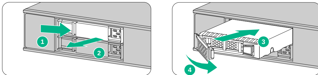
图2-14 安装硬盘
