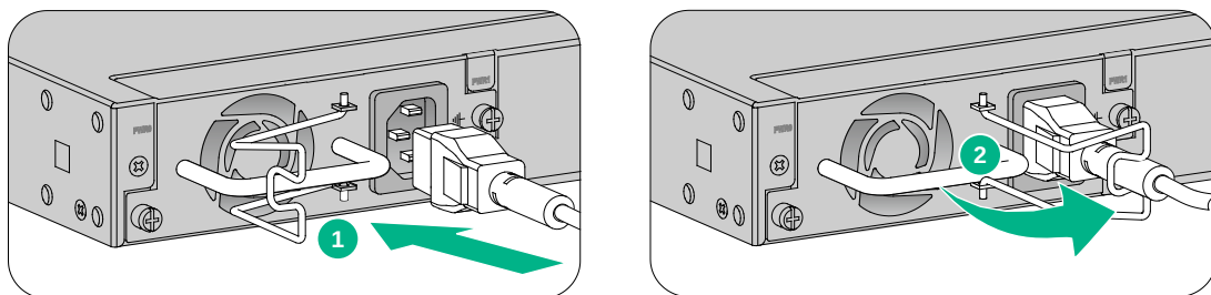
图2-19 连接交流电源线（通过卡钩的方式固定电源线）
