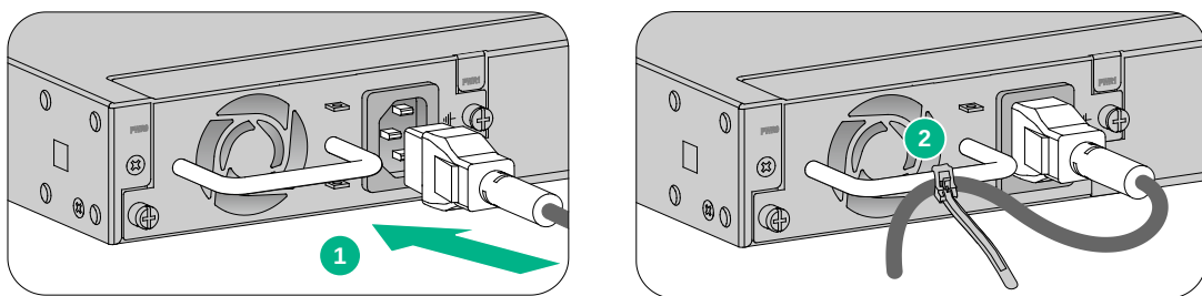
图2-20 连接交流电源线（通过扎带的方式固定电源线）
