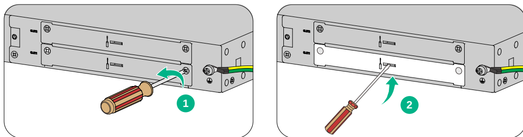
图2-12 拆卸假面板
