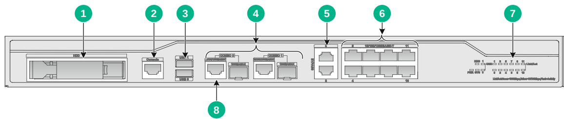
图A-1 设备前视图
