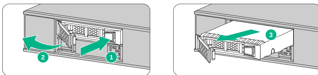
图2-15 拆卸硬盘
