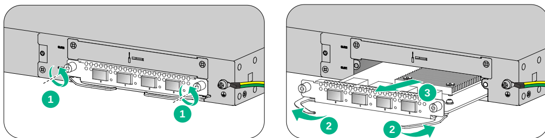
图4-2 拆卸接口模块
