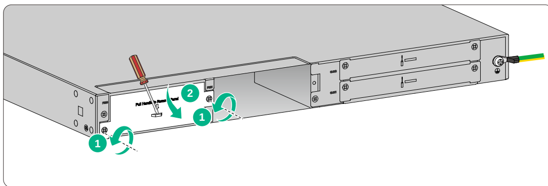
图2-10 拆卸电源假面板
