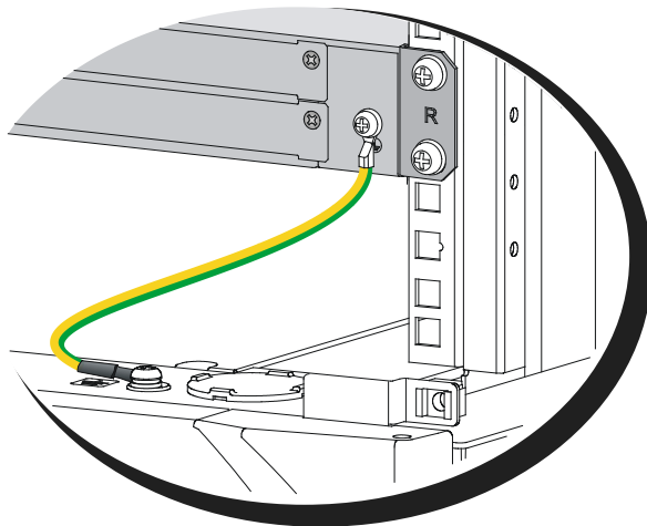
图2-9 连接到机柜接地
