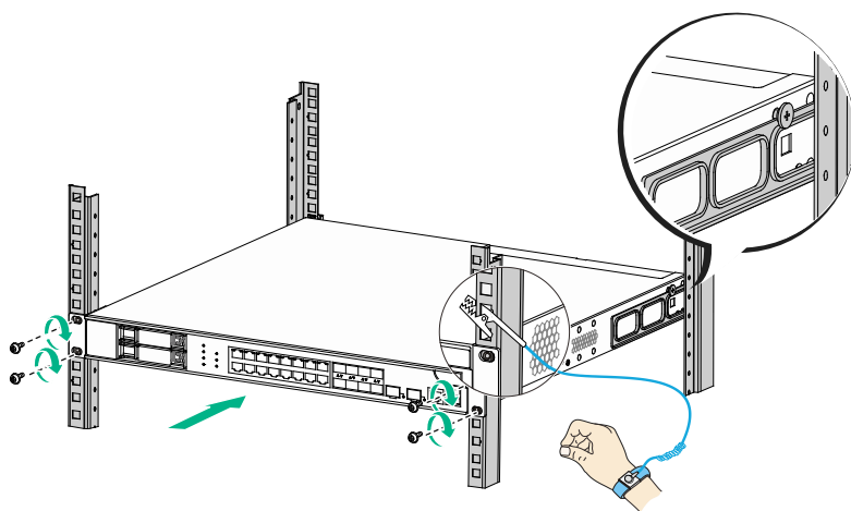
图2-6 安装设备到机柜（后挂耳正装）
