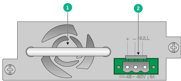
图A-12 直流电源模块外观
