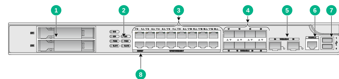
图A-7 设备前视图
