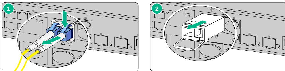
图4-4 拆卸光接口模块示意图
