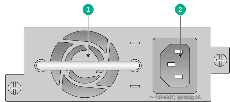
图A-11 交流电源模块外观
