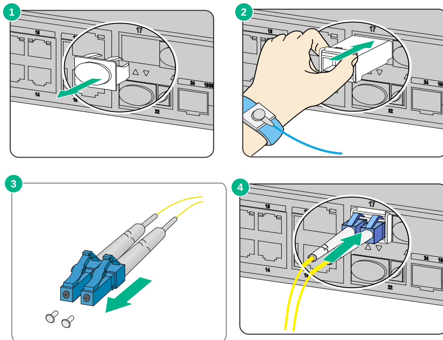
图2-18 安装及连接光模块
